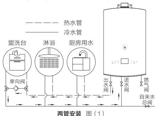
两管安装 图（1）
