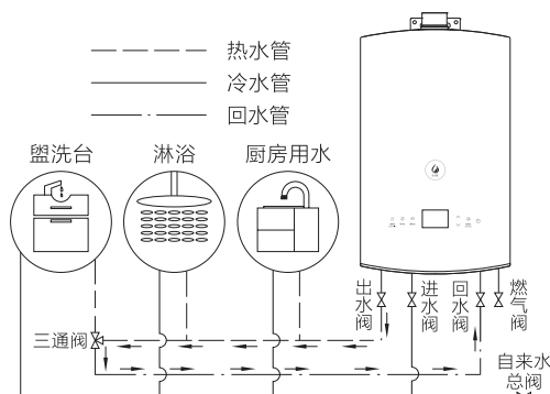
三管安装 图（2）
