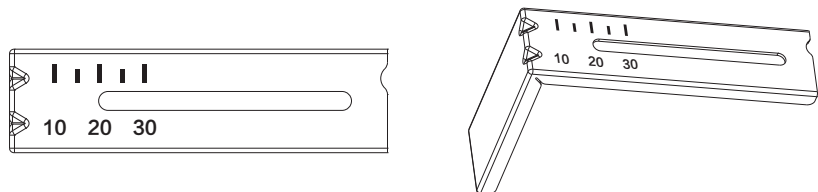
图（10）限位支架示意图
