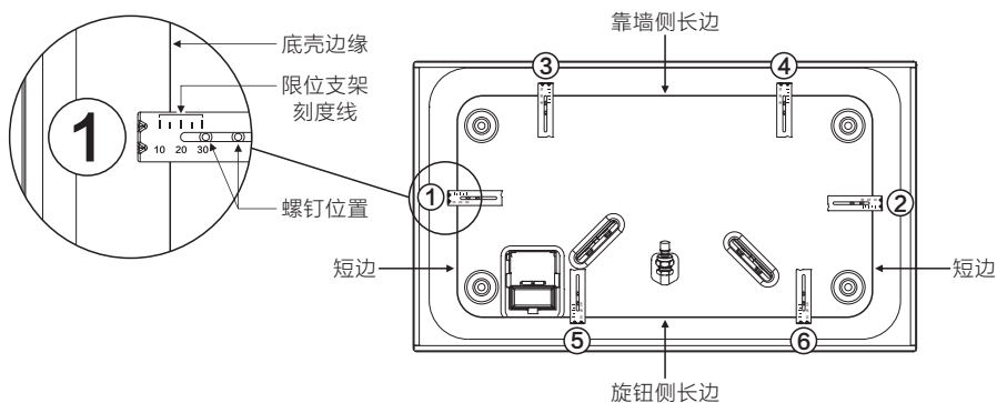
图（11）限位支架安装位置示意图
